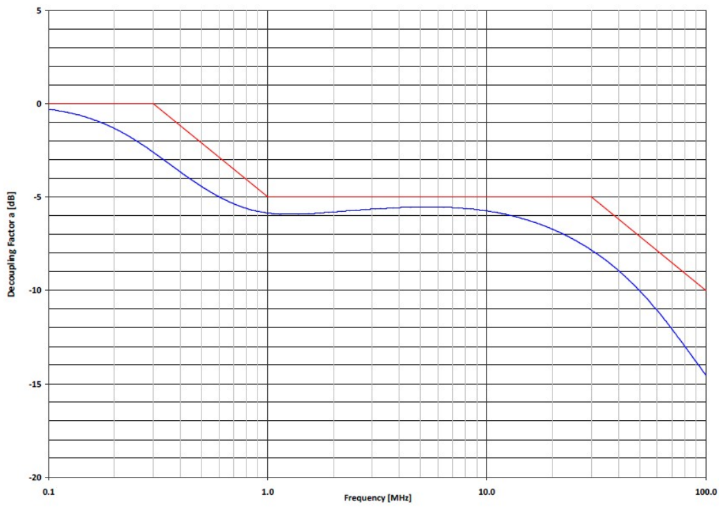
典型去耦因子
