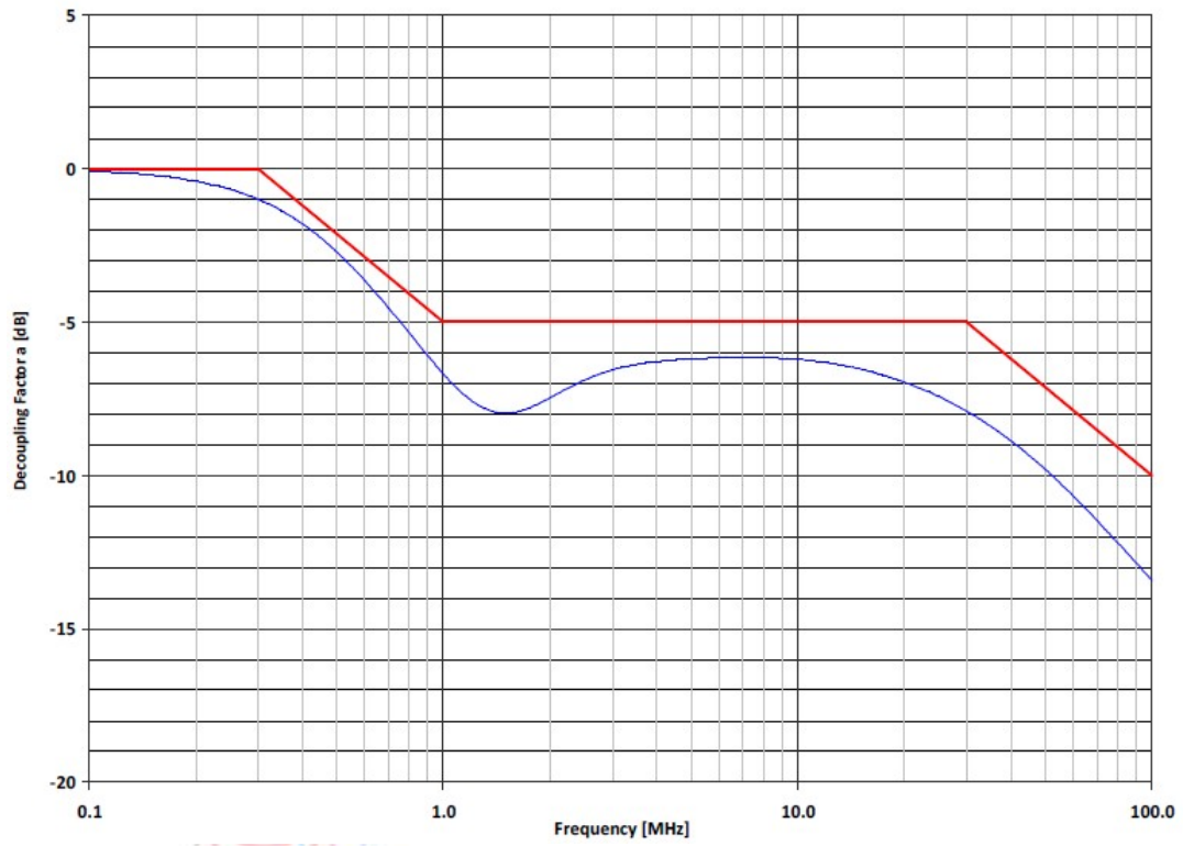
典型去耦因子
