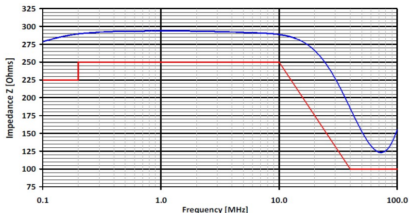
典型阻抗
