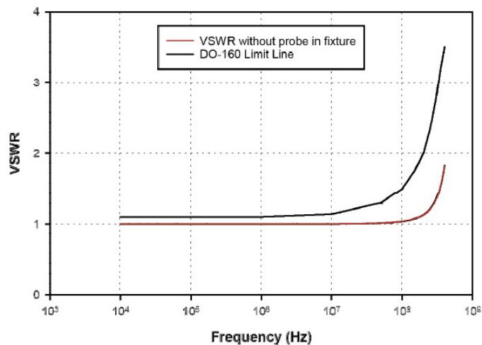
典型 VSWR
