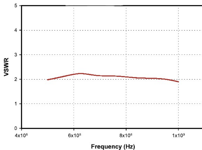
典型 VSWR
