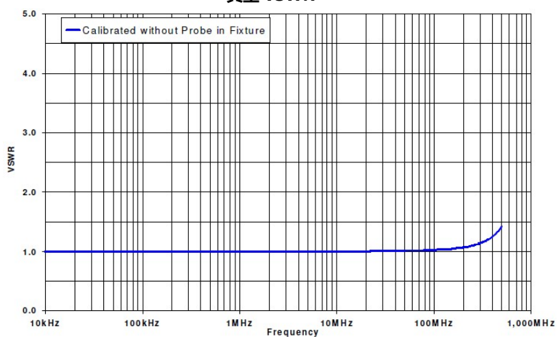
典型 VSWR
