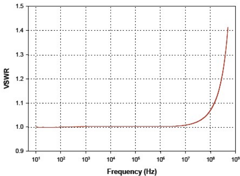
典型 VSWR
