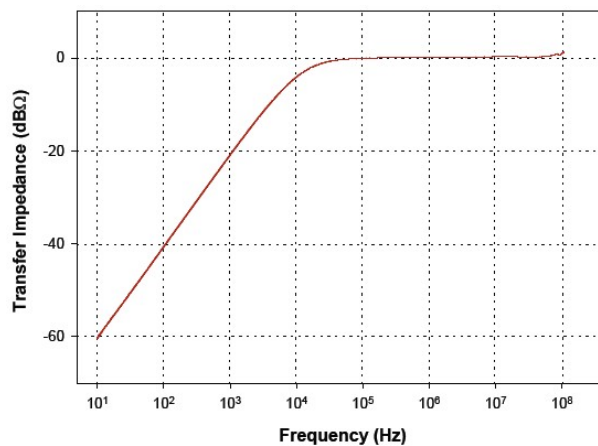
典型传输阻抗
