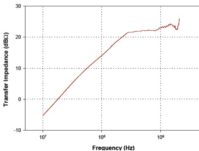
典型传输阻抗
