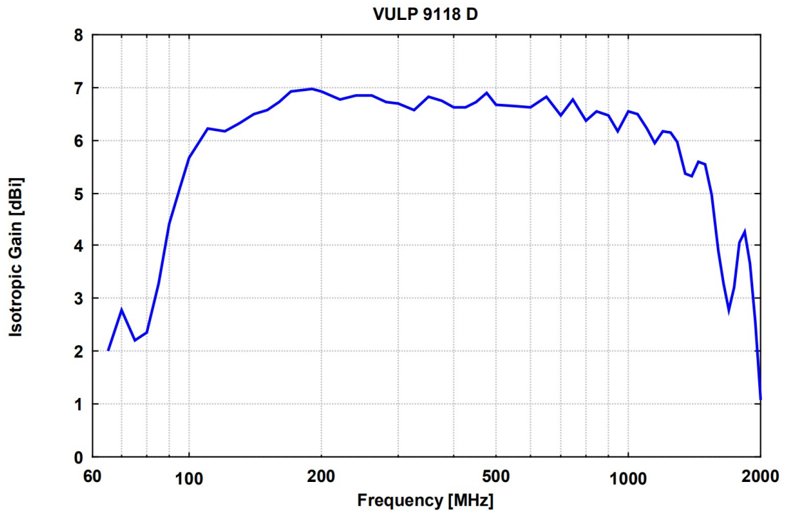
增益
