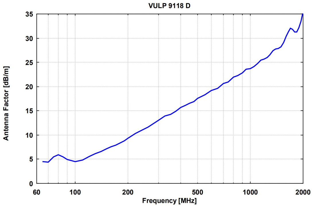
天线因子
