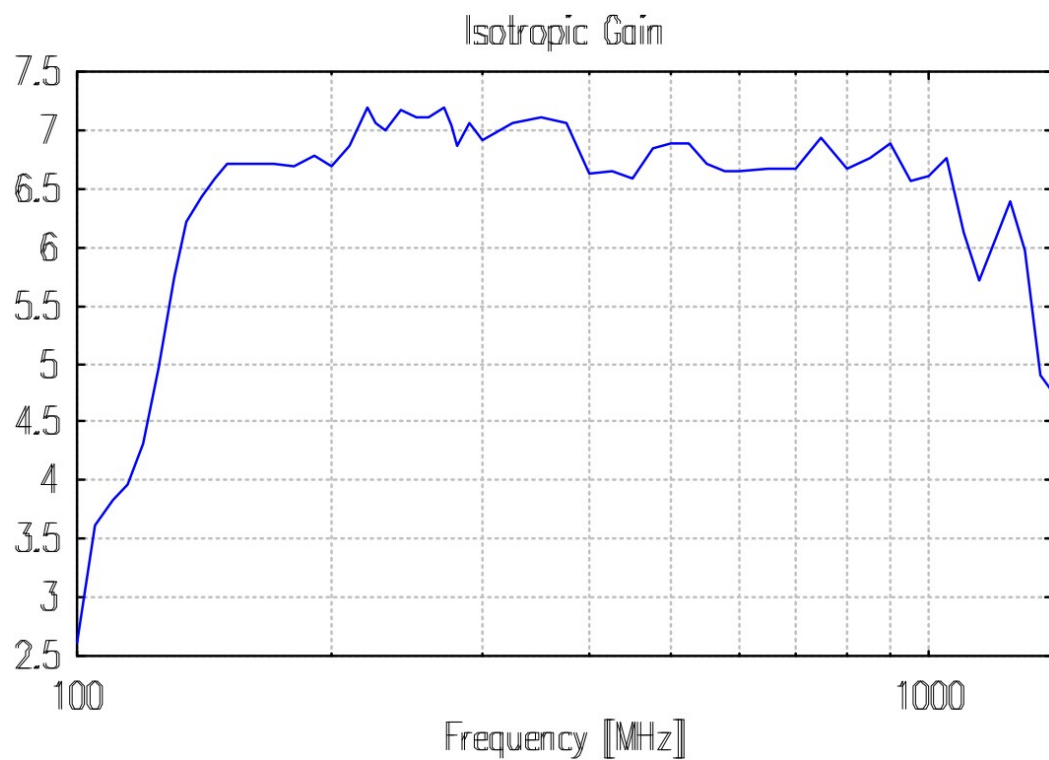
增益
