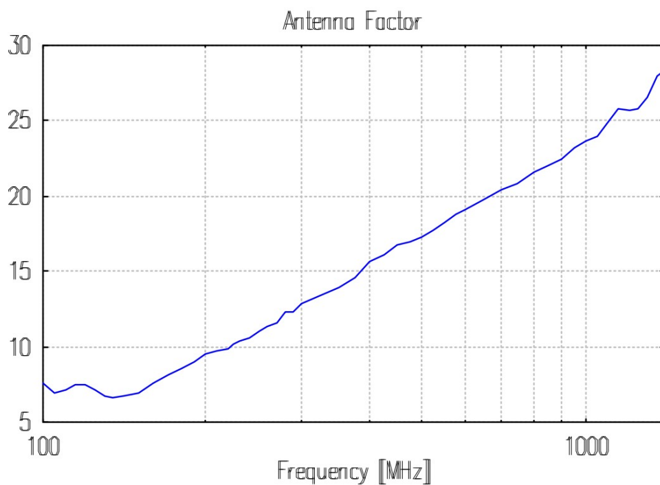
天线因子
