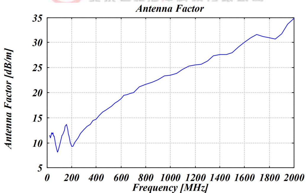
天线因子
