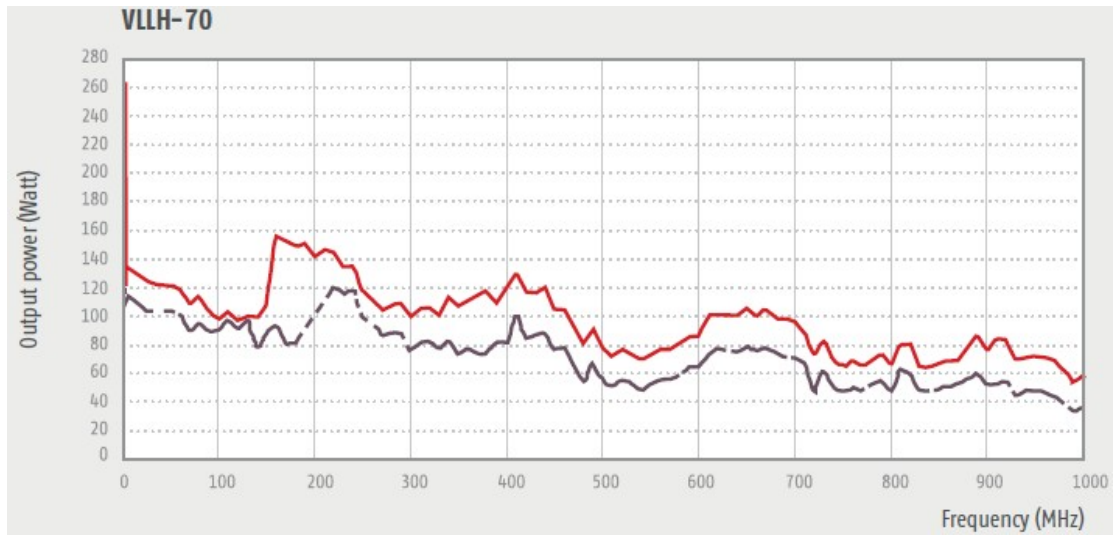
VLLH-70----- 1dB/—— 3dB 压缩点输出功率
