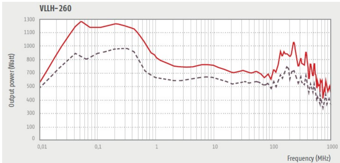
VLLH-260----- 1dB/—— 3dB 压缩点输出功率
