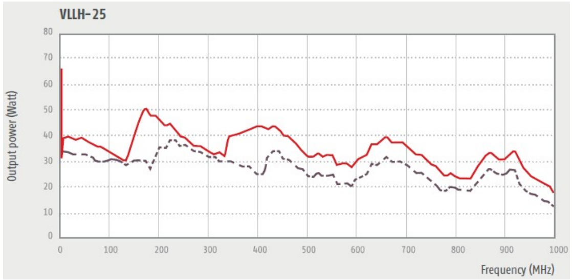
VLLH-25----- 1dB/—— 3dB 压缩点输出功率
