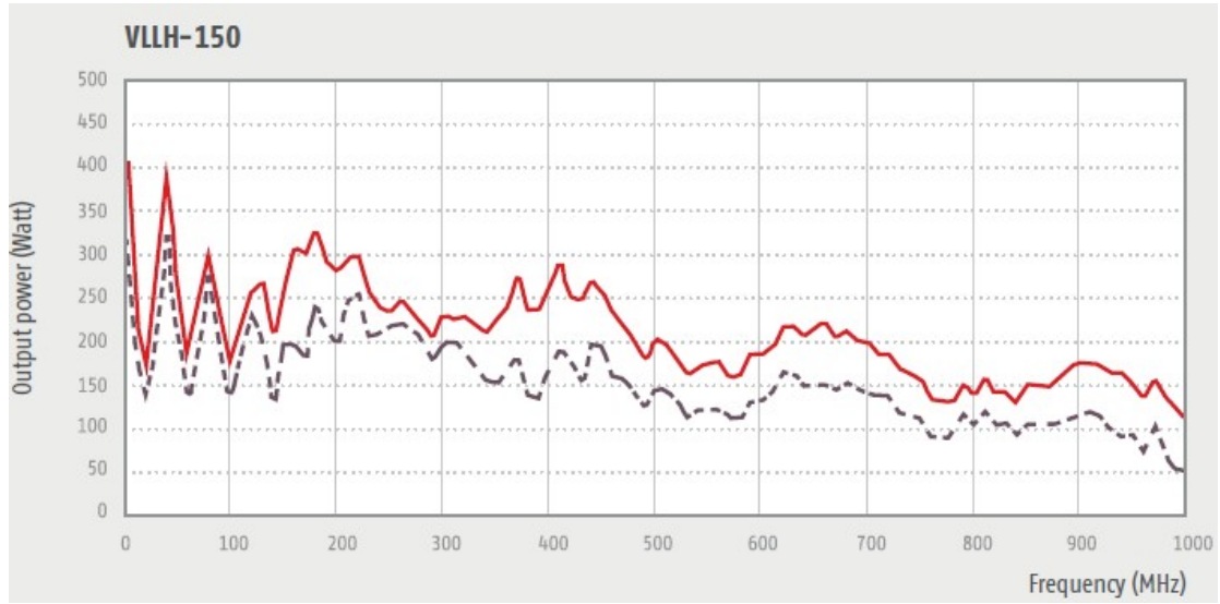
VLLH-150----- 1dB/— 3dB 压缩点输出功率
