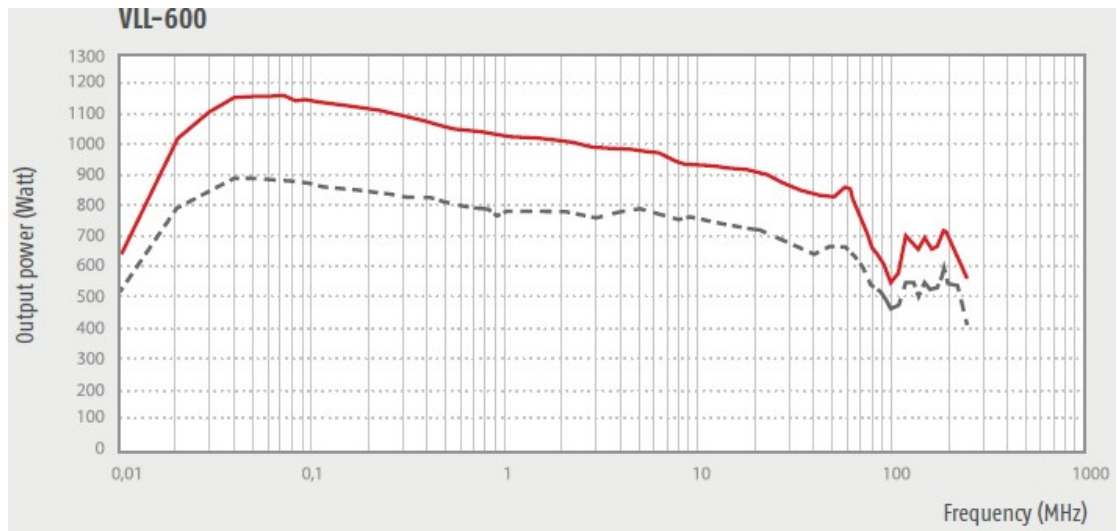
VLL-600----- 1dB/—— 3dB 压缩点输出功率
