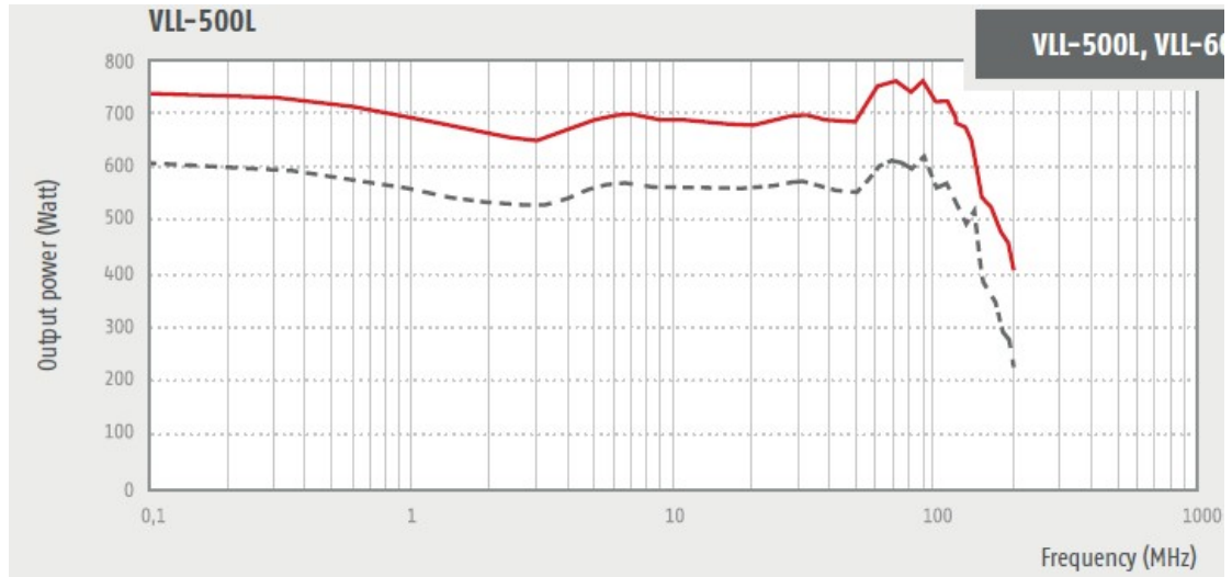
VLL-500L----- 1dB/—— 3dB 压缩点输出功率
