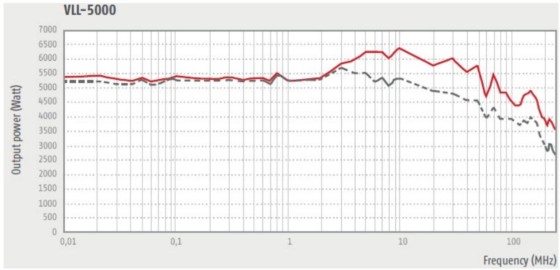
VLL-5000----- 1dB/—— 3dB 压缩点输出功率
