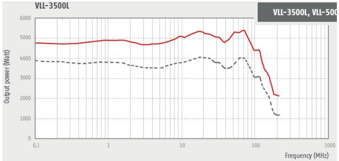
VLL-3500L----- 1dB/—— 3dB 压缩点输出功率
