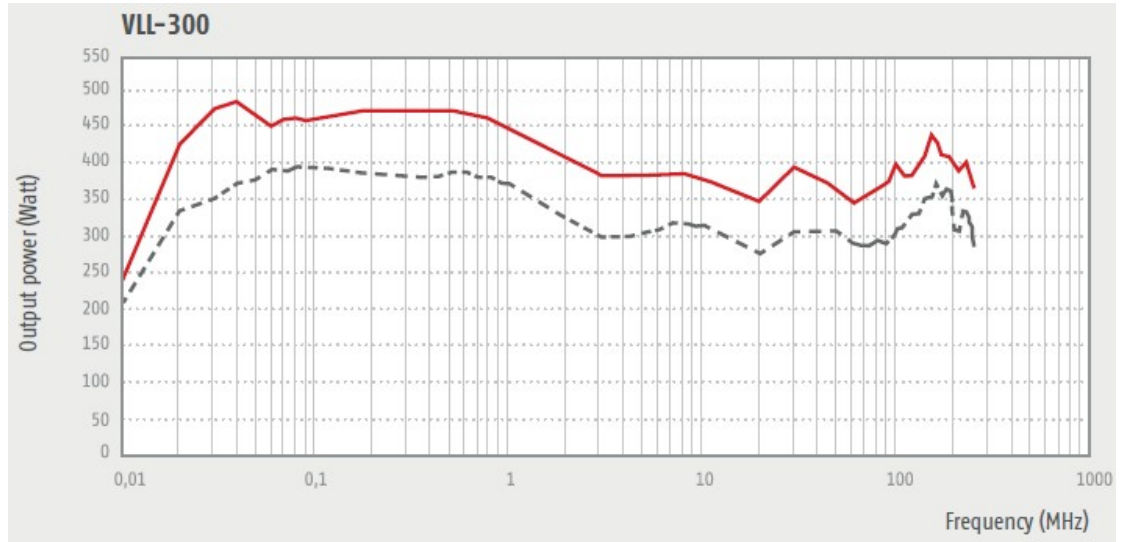
VLL-300----- 1dB/—— 3dB 压缩点输出功率
