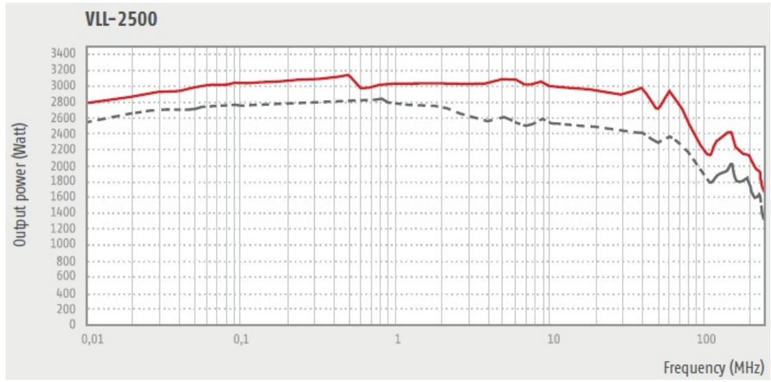
VLL-2500----- 1dB/—— 3dB 压缩点输出功率
