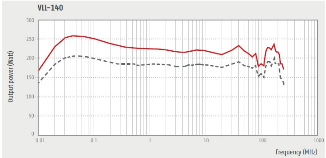
VLL-140----- 1dB/—— 3dB 压缩点输出功率
