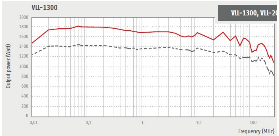
VLL-1300----- 1dB/—— 3dB 压缩点输出功率
