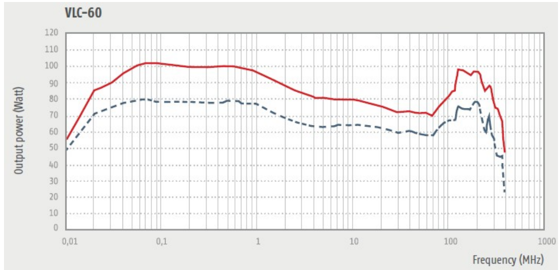
VLC-60----- 1dB/—— 3dB 压缩点输出功率
