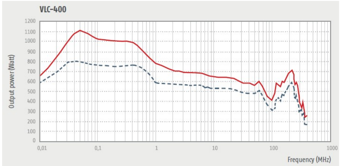
VLC-400----- 1dB/—— 3dB 压缩点输出功率
