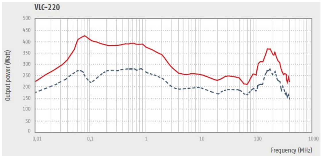
VLC-220----- 1dB/—— 3dB 压缩点输出功率
