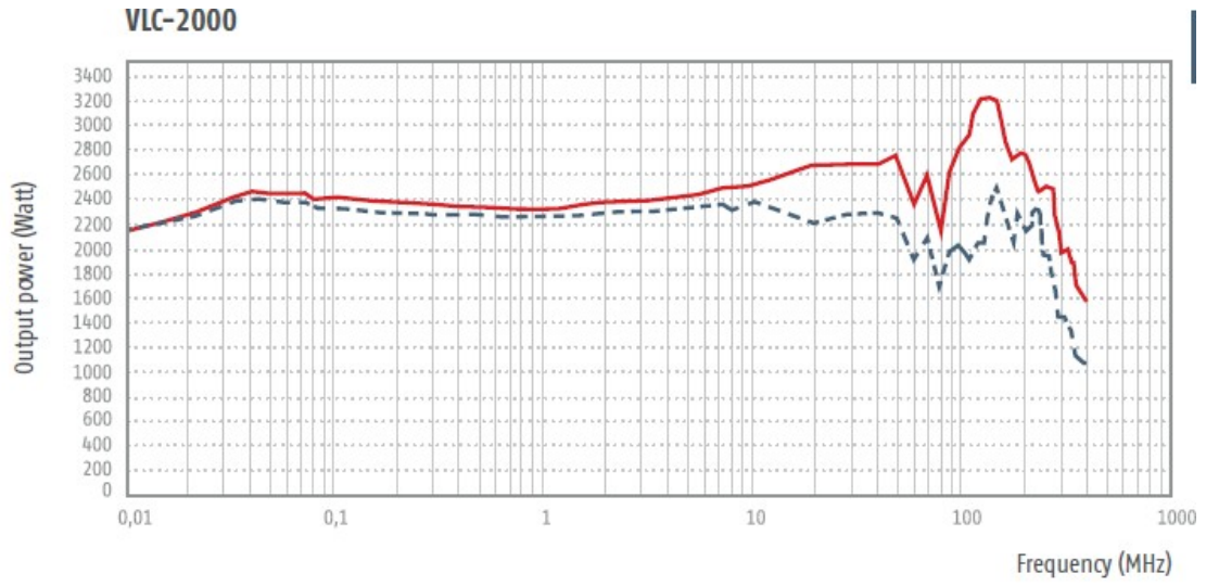
VLC-2000----- 1dB/—— 3dB 压缩点输出功率
