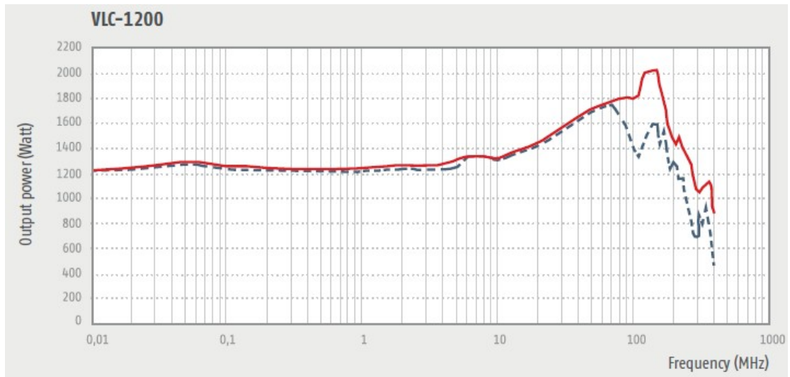
VLC-1200----- 1dB/—— 3dB 压缩点输出功率
