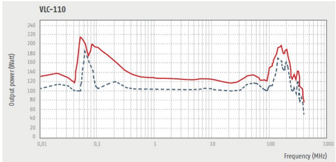
VLC-110----- 1dB/—— 3dB 压缩点输出功率
