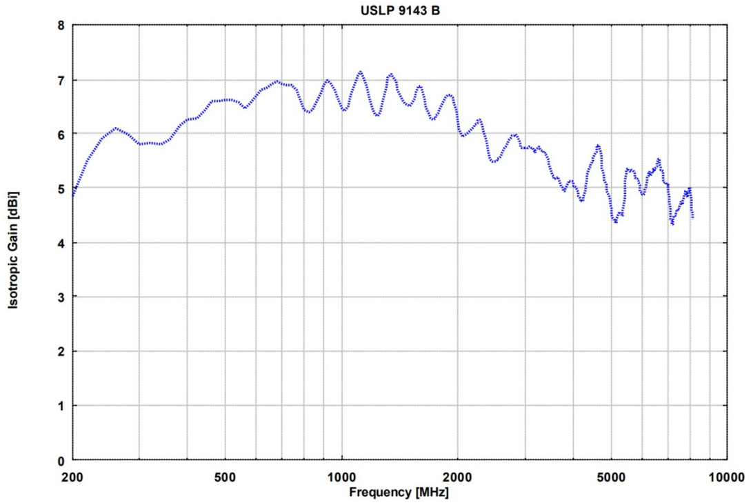
增益
