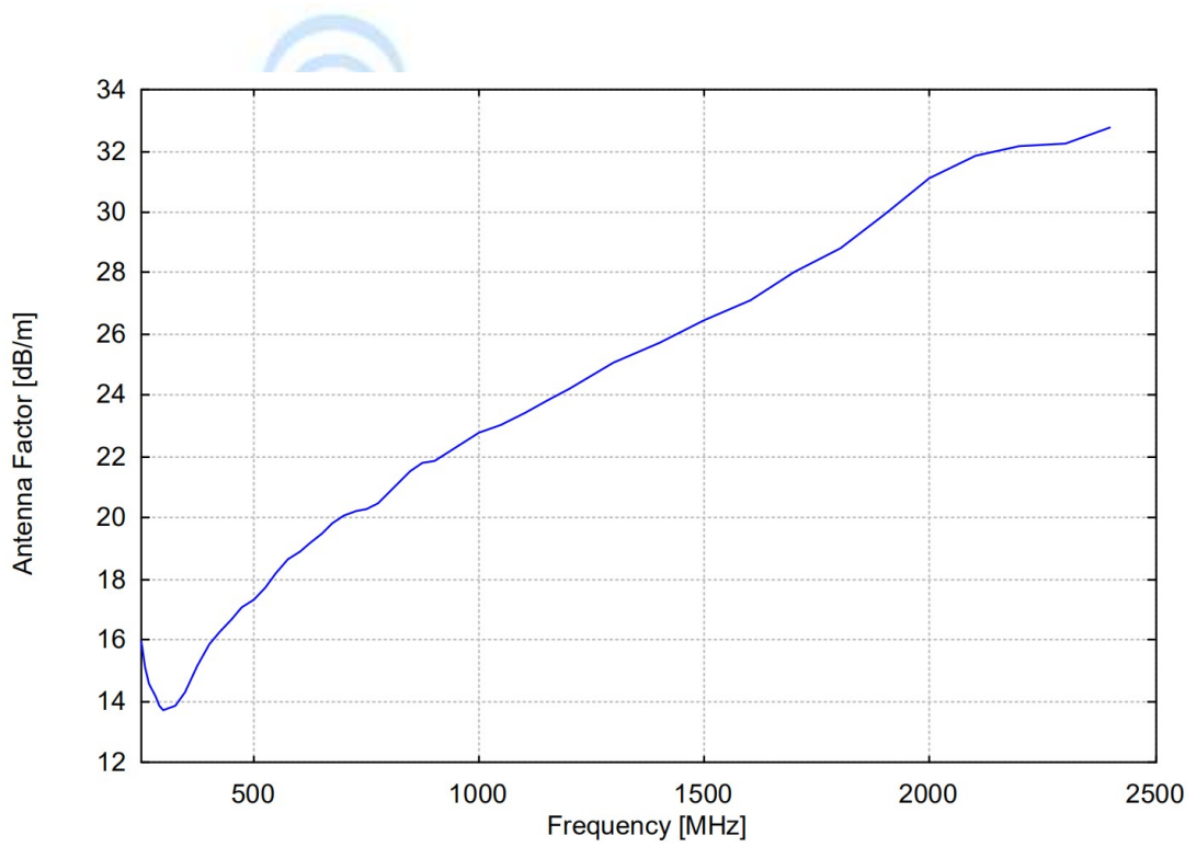
天线因子
