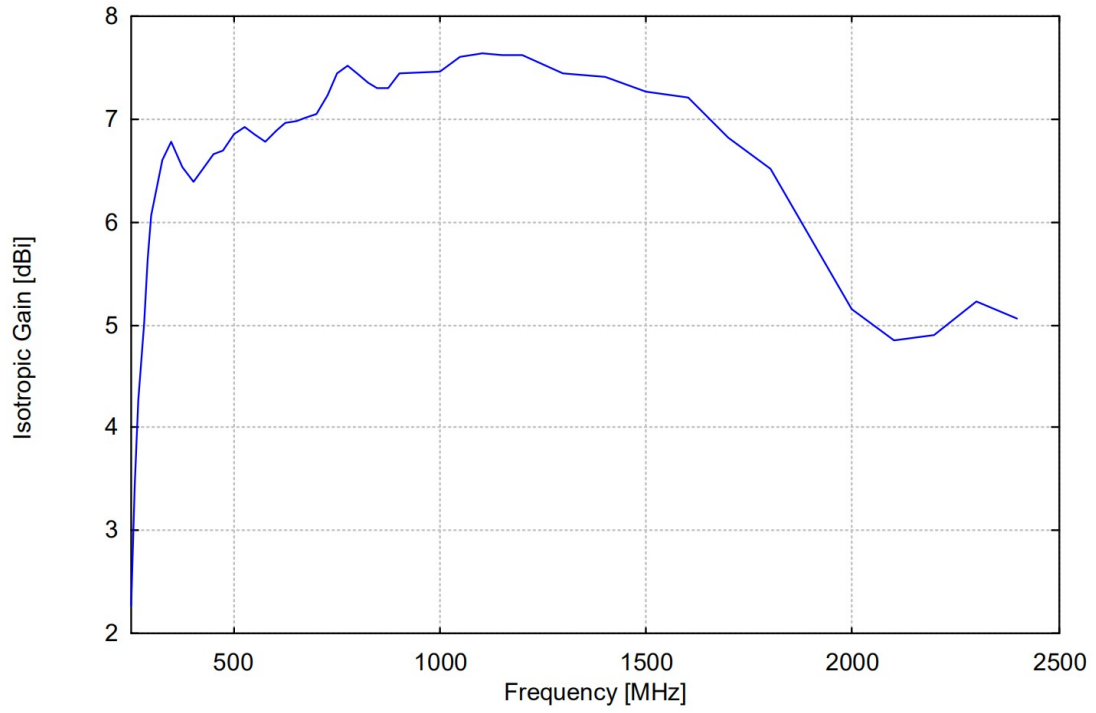
增益
