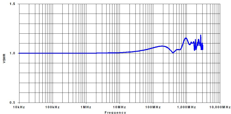
典型 VSWR
