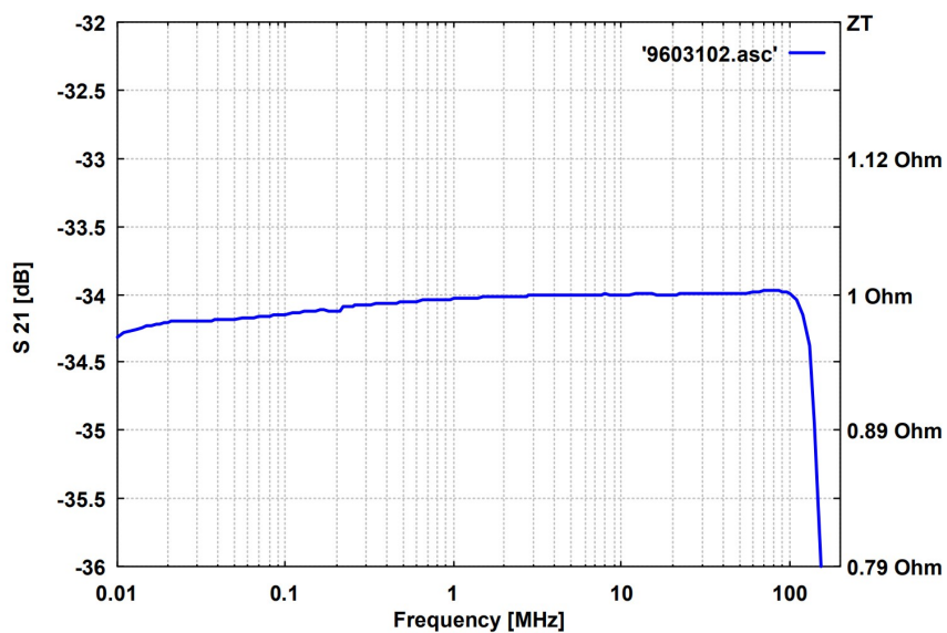
50 欧姆系统的传输阻抗
