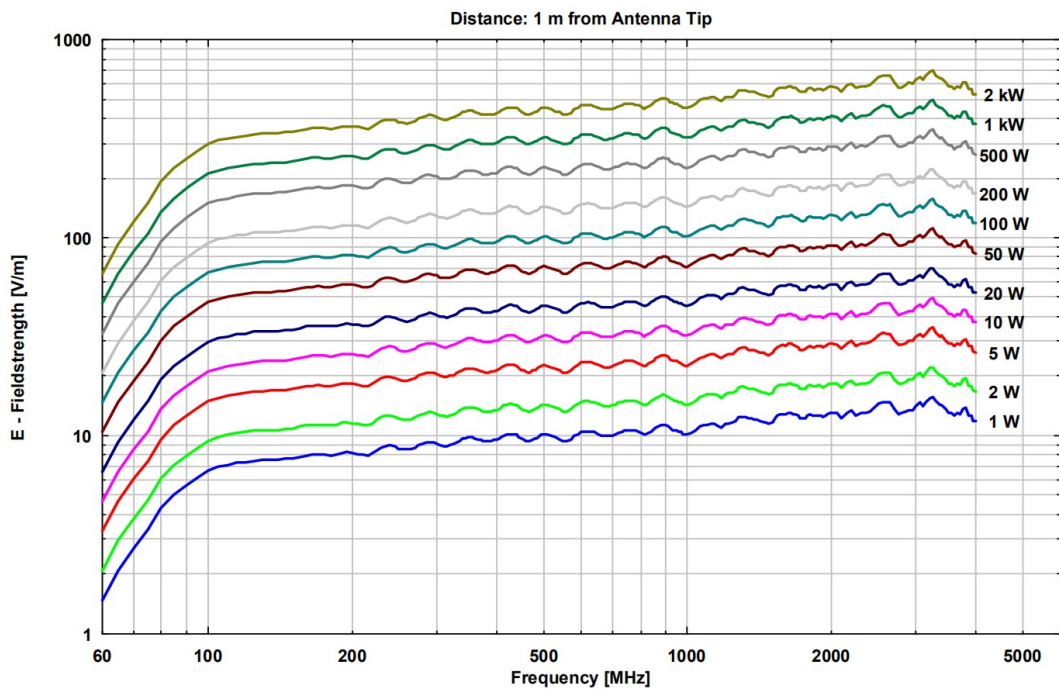
功率与场强 (测试距离: 1 米)
