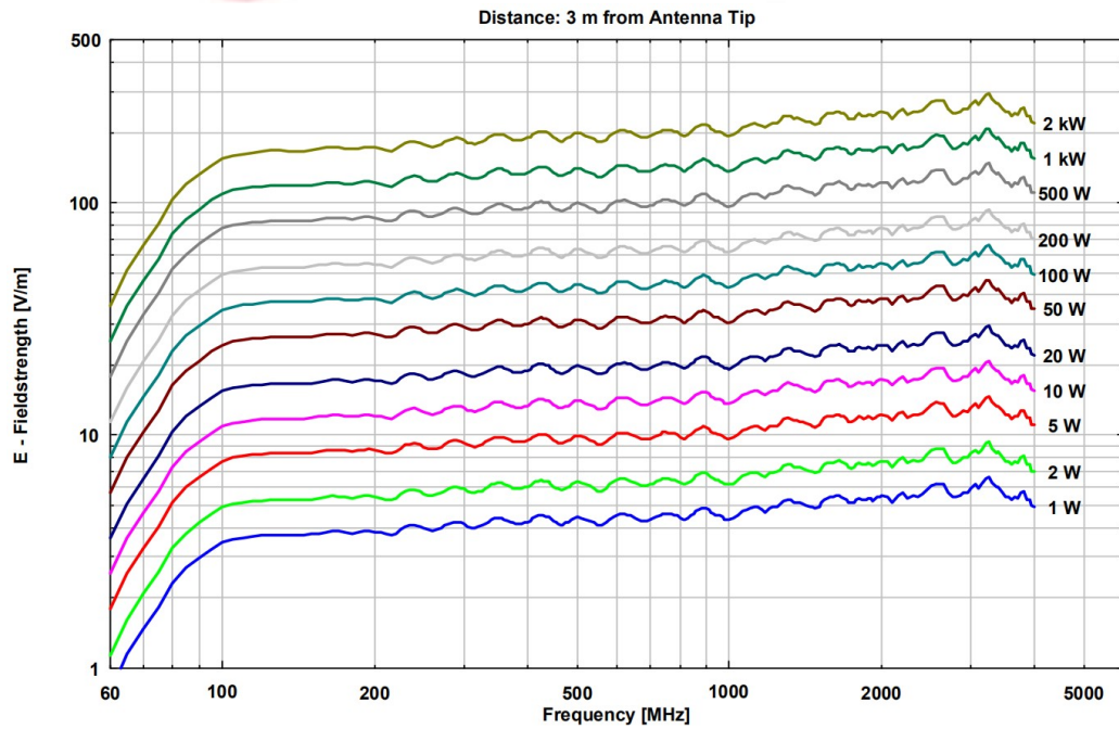
功率与场强 (测试距离: 3 米)
