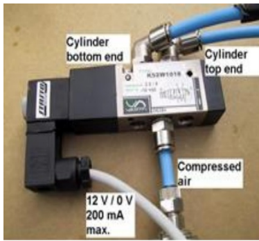
转向电磁阀连接
