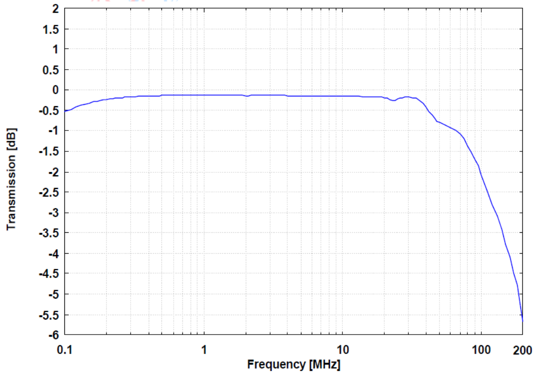
分压系数比, EuT 端子到 N 连接器 (需要适配器)
