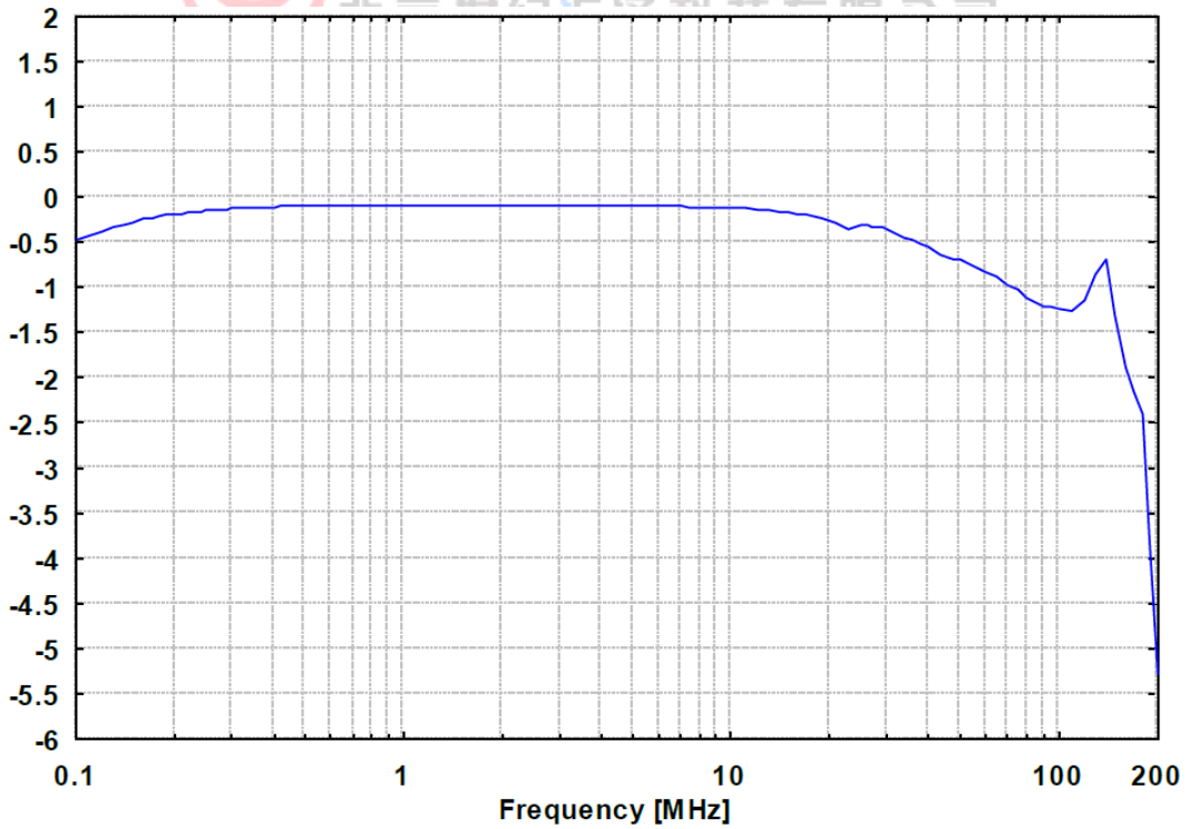
阻抗特性曲线
