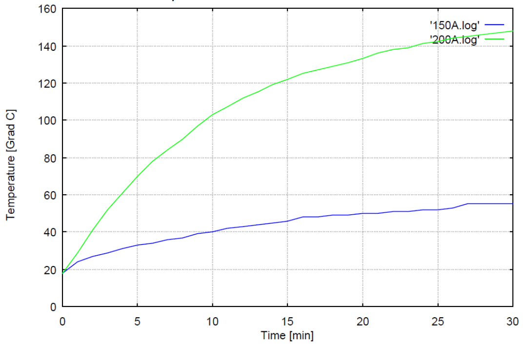
连续电流下的温升特性
