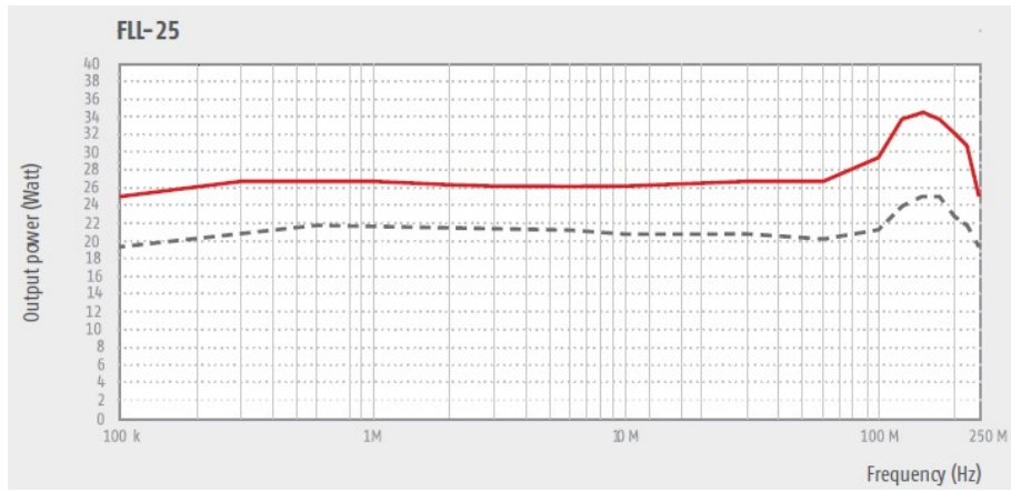
FLL-25----- 1dB/—— 3dB 压缩点输出功率
