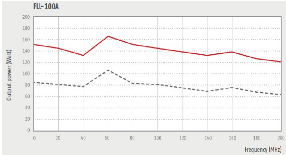
FLL-100A----- 1dB/—— 3dB 压缩点输出功率
