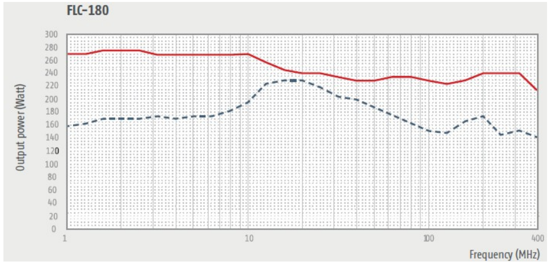
FLC-180----- 1dB/—— 3dB 压缩点输出功率
