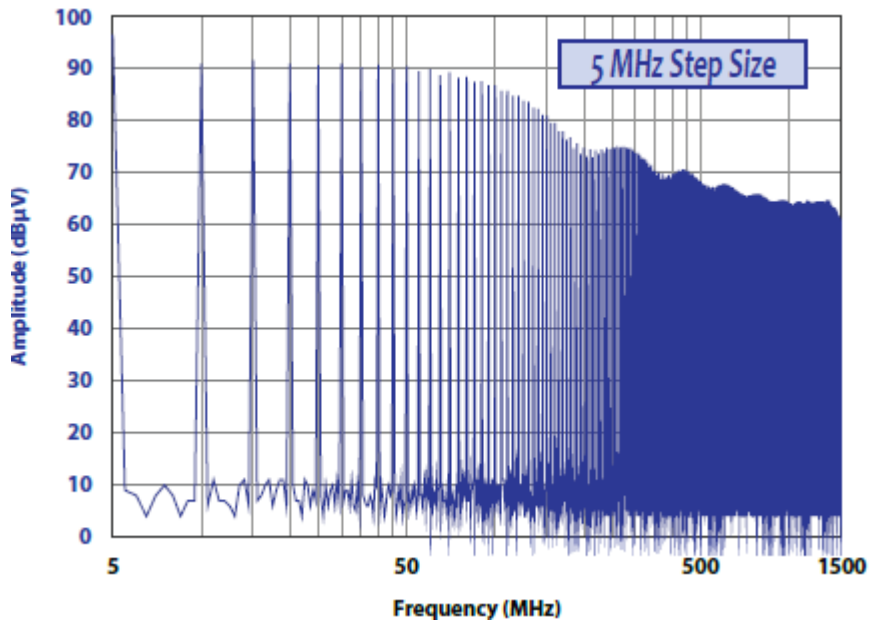
传导发射, 5MHz 步长
