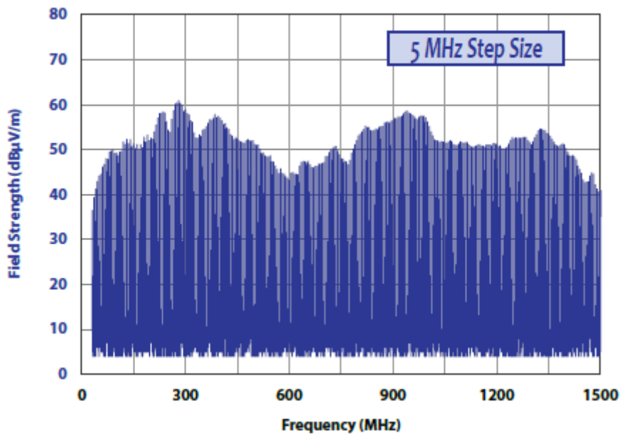
辐射发射，5MHz 步长
