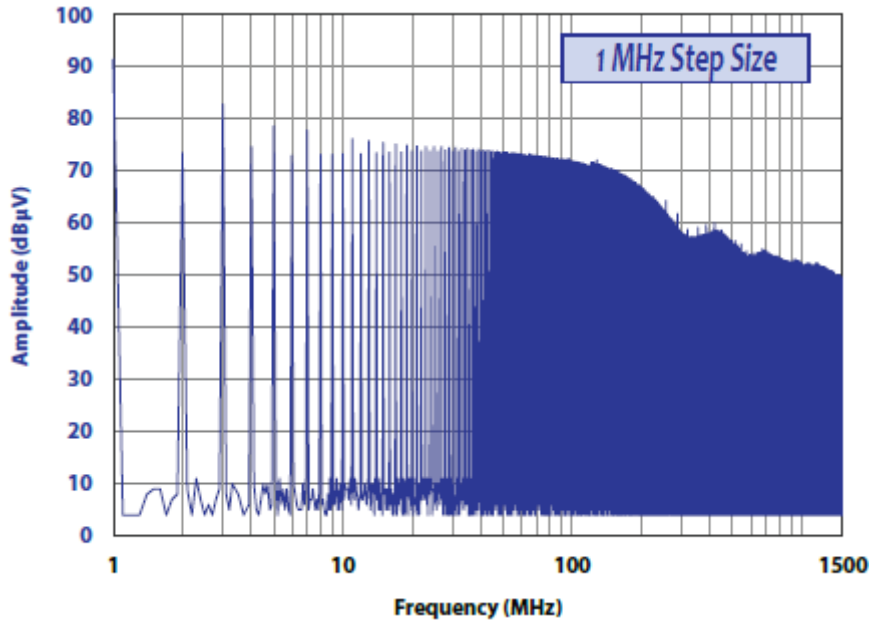
传导发射, 1MHz 步长
