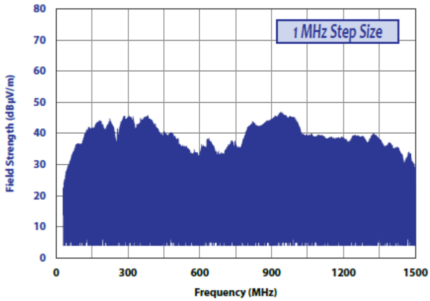
辐射发射，1MHz 步长
