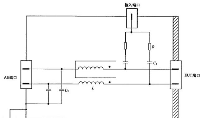
用于非屏蔽不平衡线的耦合去耦网络 CDN-AF2 电路图
