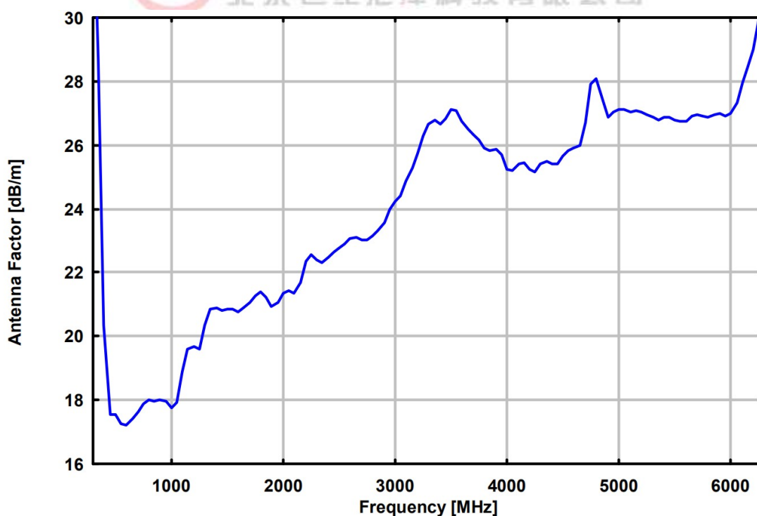
天线因子
