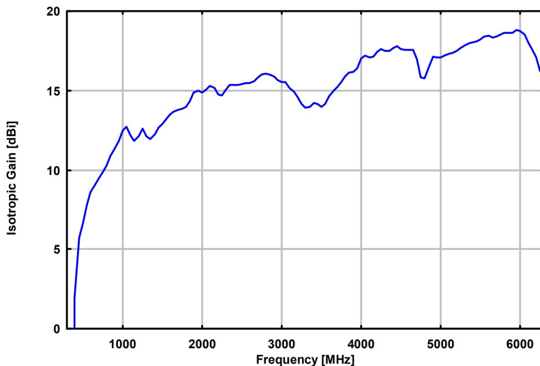
增益
